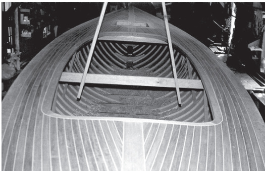
Däcket färdigputsat
