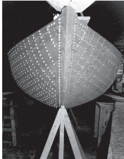
Bordläggningen proppad
