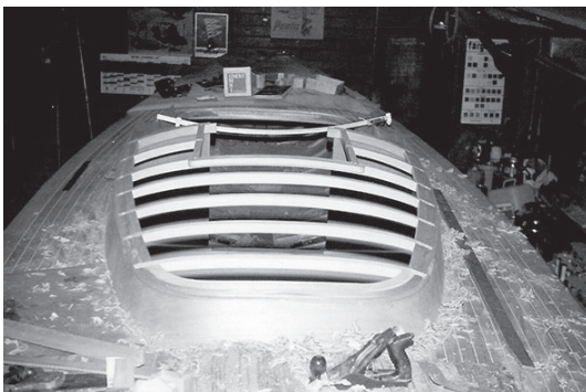
Klart för att lägga rufftaket Däck, skarndäck, livrä och mittfisk på plats
