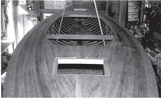
Däck, skarndäck, livrä och mittfisk på plats
